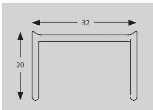
Ladenführungsprofil Art. 8017
