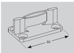
Bodenführung Art. 8022
