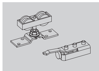
Laufwagen Art. 8020 Schienenpuffer Art. 8021
