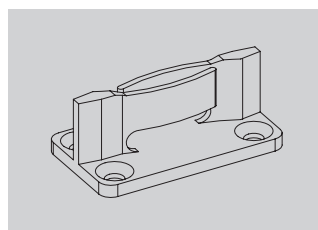
Bodenführung Art. 8022
