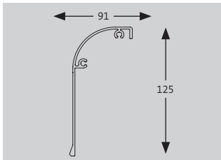
Abdeckblende Art. 8104
