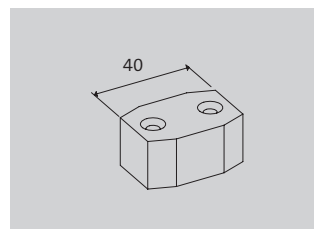
Untere Führung Art. 8046
