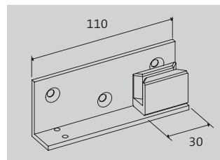
Untere Führung Art. 8043
