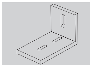
Winkel Doppelflügel Art. 8003
