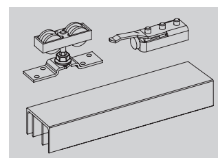
Schiebeladen-Set Art. 8000
