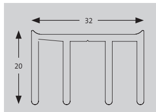
Ladenführungsprofil Art. 8018
