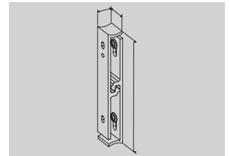
Mittelverschluss Art. 5805
