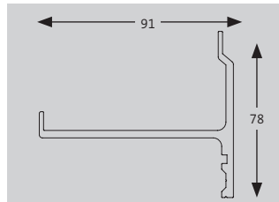
Trägerprofil Art. 8107
